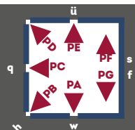
Schweißpositionen nach EN 287 und ISO 6947
