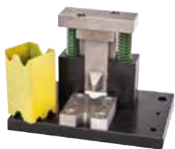
Keilformige Stanze
