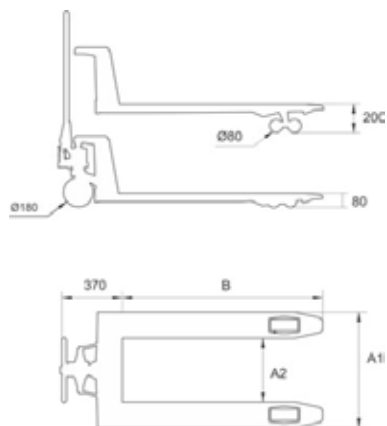
Abmessungen: A2 = 240 mm
