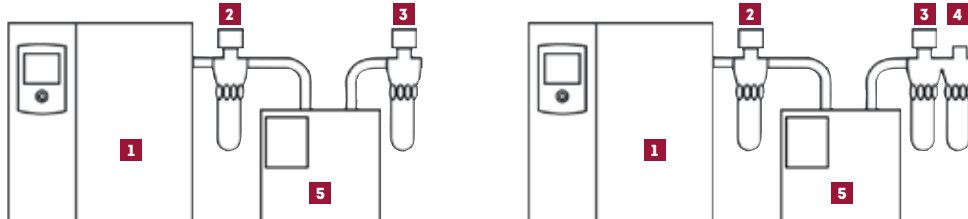
Qualitätsdruckluft mit niedrigerem Taupunkt (Luftreinheit nach ISO 8573-1: Klasse 1:4:2)
