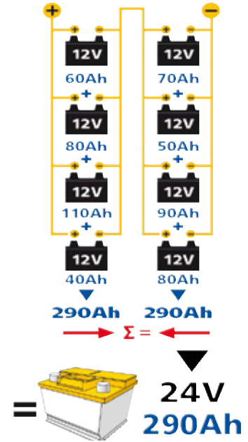
Kombination zwischen Parallel- & Serienschaltung
