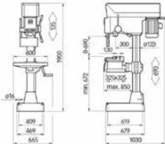
R40E PGM
