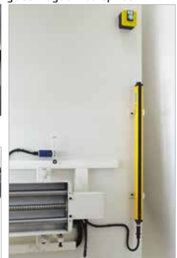
Rückseite: Lichtschranke mit Prüfeinrichtung
