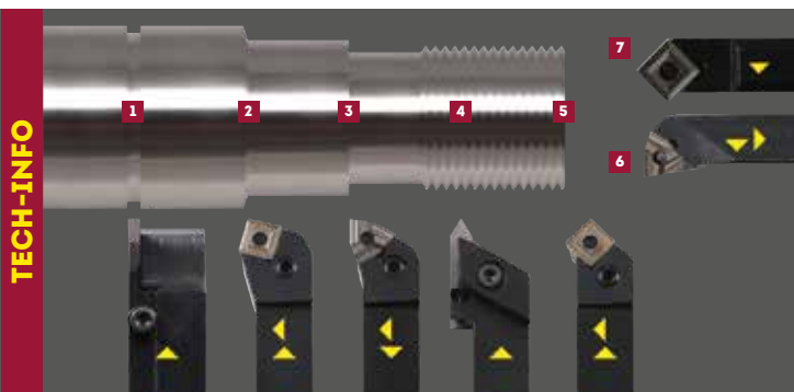
Drehmeißelformen und -funktionen
