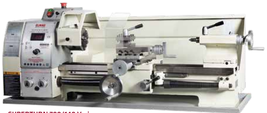
SUPERTURN 700/140 Vario
