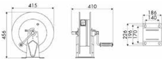
Abmessungen Modelle 74300/10, 74320/10, 74340/20, 74340/30, 74305/10, 74345/30
