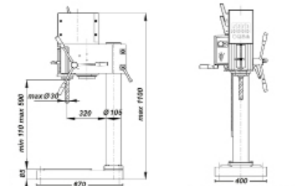
Tischbohrmaschine
