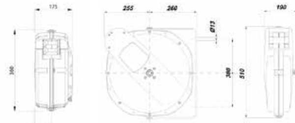
Abmessungen des Modells INDUSTRIE 21
