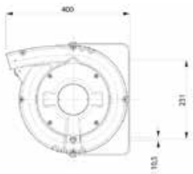
Abmessungen des Modells INDUSTRIE 12
