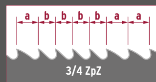
Beispiel für variable Zahnteilung 3/4 ZpZ:
