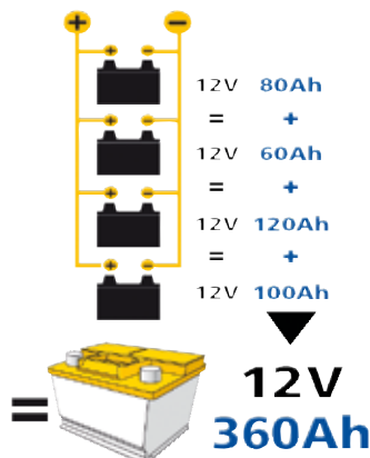
Parallelschaltung
