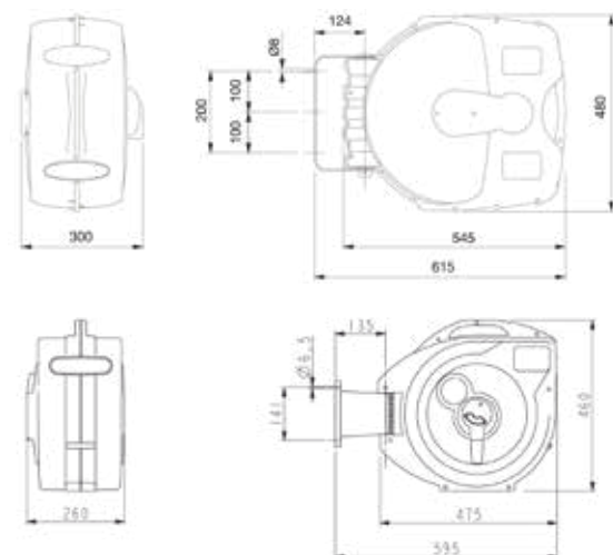
Abmessungen Modelle MEGA
