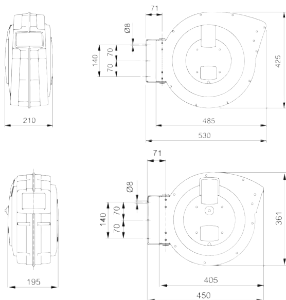
Abmessungen der Modelle MEGA 230 u. 400
