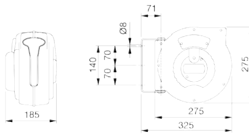
Abmessungen des Modells JUNIOR 9
