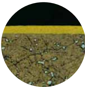
Mikroskop-Bild der Hartstoffschicht des TiN beschichteten Sägeblattes
