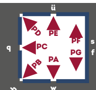
Schweißpositionen nach EN 287 und ISO 6947
