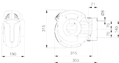
Abmessungen des Modells MASTER 12
