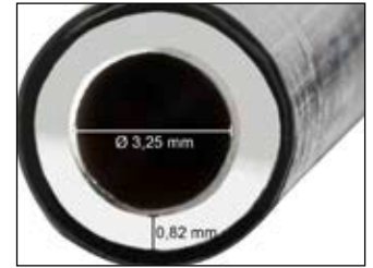
Neuartige Bremsleitung
